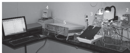
Figura 1 - Sistema de perfusão pulmonar isolada denominado IL-2 Isolated Perfused Rat or Guinea Pig Lung System . 1) câmara de pressão negativa; 2) bomba de perfusão de roletes conectada; 3) reservatório de sangue e desoxigenador de membrana; 4) aquecedor de água com circulação em torno de todo o sistema de perfusão para a manutenção de temperatura; e 5) módulo de aquisição de dados hemodinâmicos, mecânica ventilatória e hemogasometria (pH, PaO 2 ) com transdutores e ventilador volumétrico acoplados a um computador pessoal.
