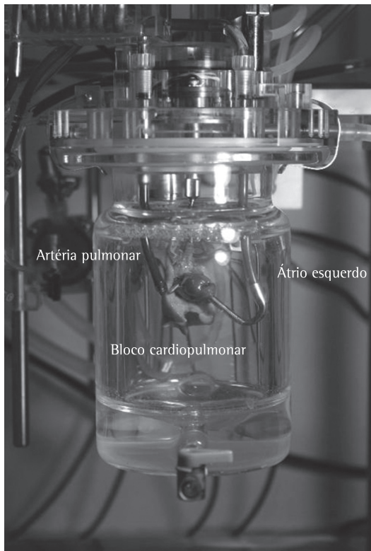
Figura 2 - Câmara de pressão negativa contendo o bloco cardiopulmonar. O bloco cardiopulmonar é posicionado na câmara de pressão negativa, conectado à ventilação, sendo perfundido pela cânula arterial pulmonar com drenagem pela cânula atrial esquerda.
